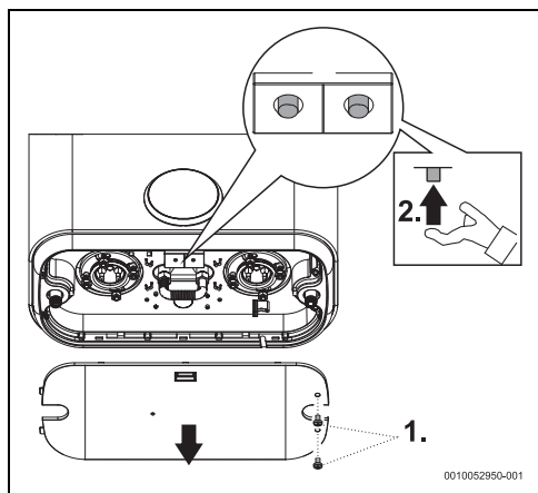
Fig. 16 Termostatos de segurança
