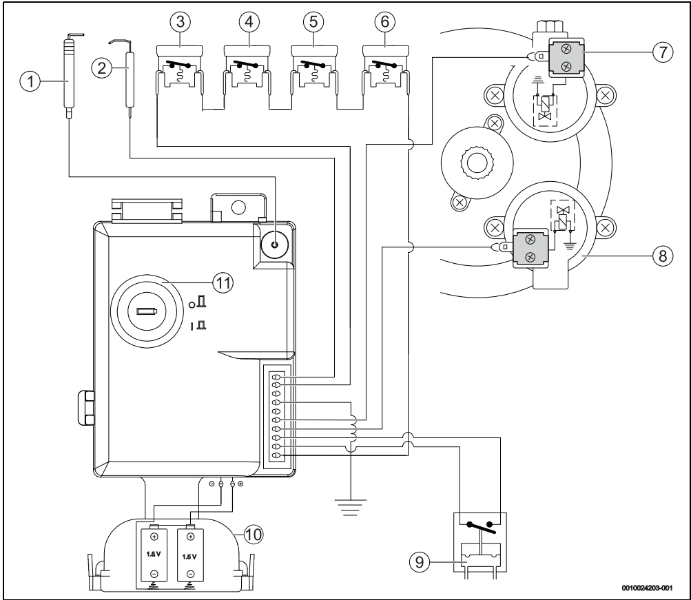
Fig. 33 Esquema elétrico
