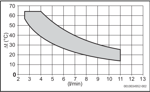
Fig. 35 Modelo 11 litros
