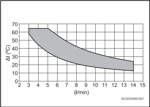
Fig. 36 Modelo 14 litros
