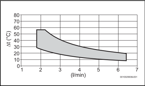
Fig. 34 Modelo 5 litros
