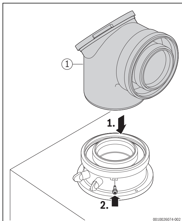
Fig. 26 Colocar e fixar os acessórios de exaustão com parafusos
