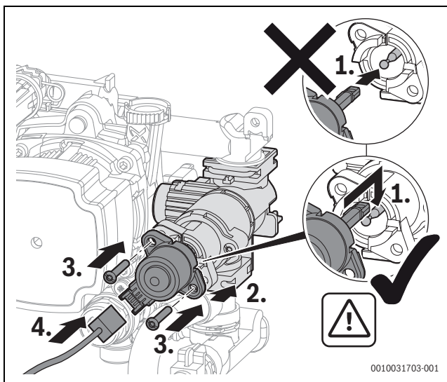
Fig. 65 Montar o motor na válvula de 3 vias (versão com parafusos)
