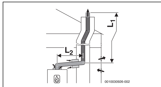
Fig. 12 Tubagem flexível de gases queimados na conduta de acordo com B_{23p}/B_{53p} com ar de admissão dependente do ar ambiente no aparelho e peça de ligação concêntrica entre o local de instalação e a conduta
