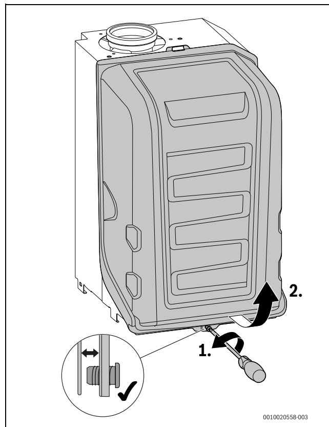
Fig. 34 Retirar a cobertura do queimador
