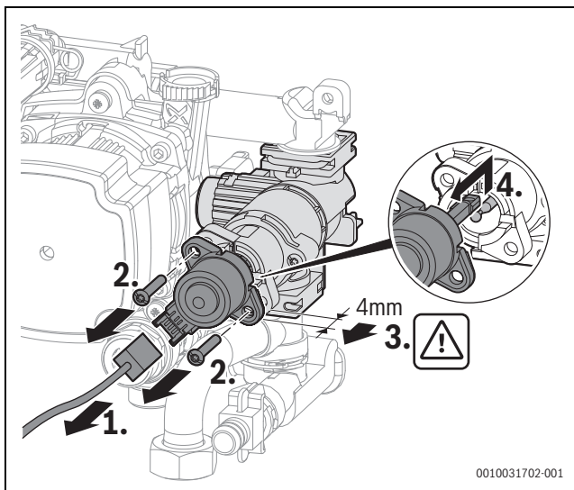
Fig. 64 Desmontar o motor na válvula de 3 vias (versão com parafusos)
