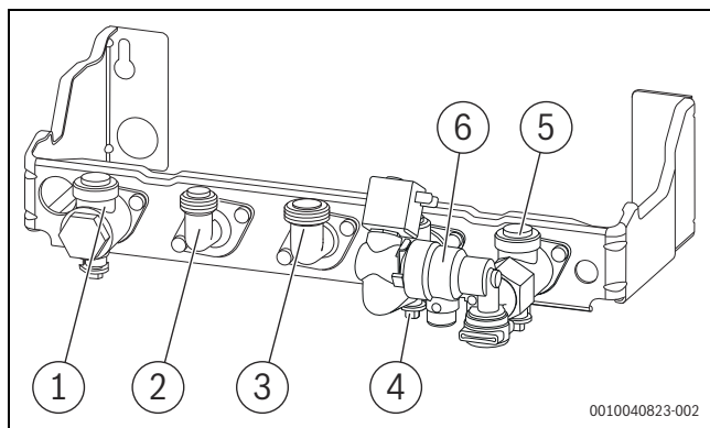
Fig. 27 Ligações do lado do gás e da água
