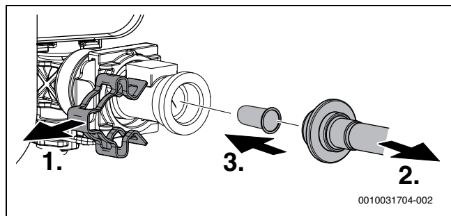
Fig. 47 Desmontar o filtro do tubo de água fria
