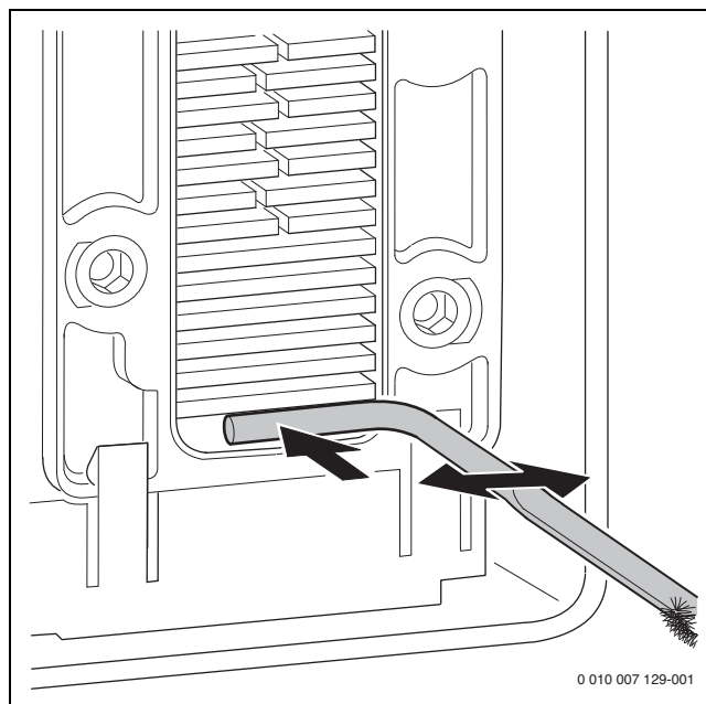
Fig. 54 Limpar a cuba de condensados
