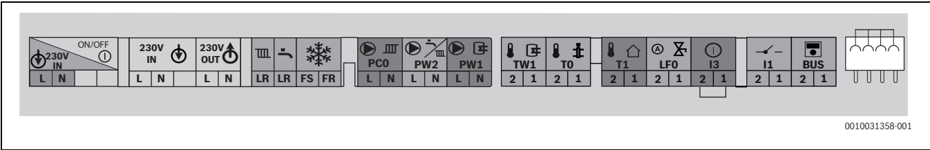
Fig. 30 Régua de bornes para os acessórios externos
