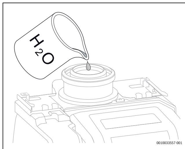
Fig. 25 Encher a recolha de condensados com água
