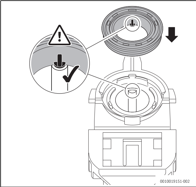
Fig. 56 Alinhar corretamente o novo vedante recolha de condensados
