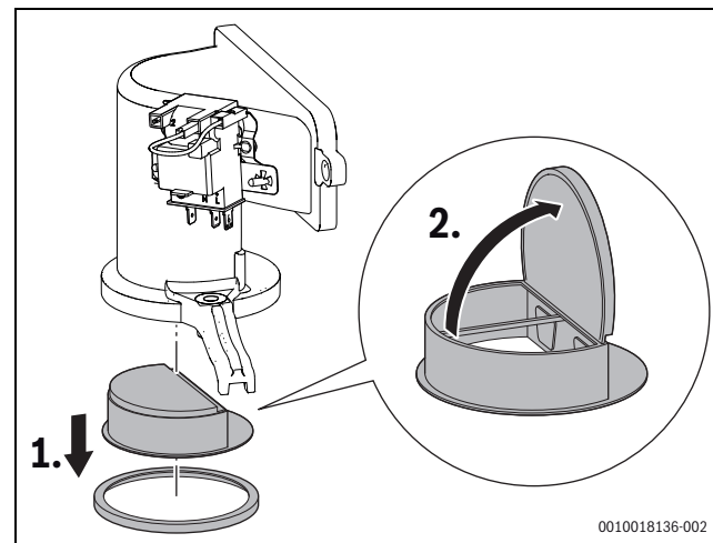
Fig. 46 Válvula antirretorno no dispositivo de mistura
