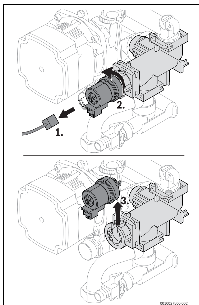
Fig. 62 Desmontar o motor na válvula de 3 vias (versão sem parafusos)
