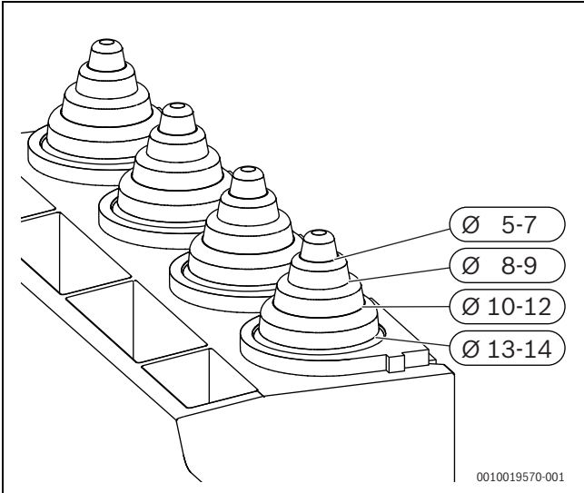
Fig. 29 Adaptar o dispositivo de redução de tração ao diâmetro do cabo
