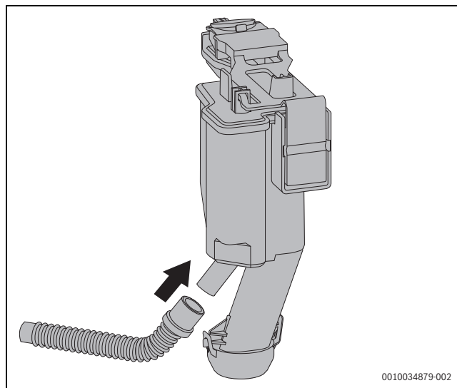
Fig. 22 Instalar a saída de condensados na placa de ligação para montagem
