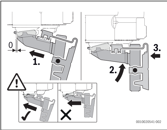
Fig. 58 Montar a recolha de condensados
