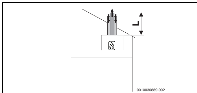
Fig. 8 Condução vertical e concêntrica dos gases de escape para o exterior de acordo com C 33x
