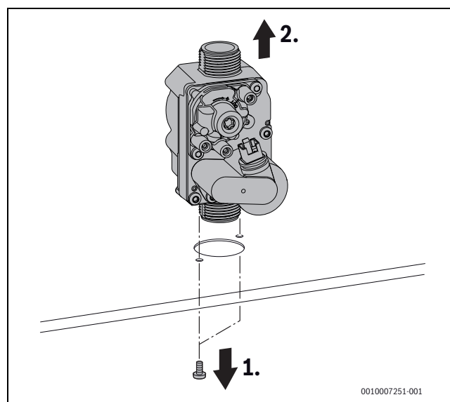
Fig. 61 Desmontar a válvula de gás
