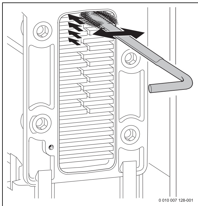
Fig. 52 Limpar o bloco térmico com a escova
