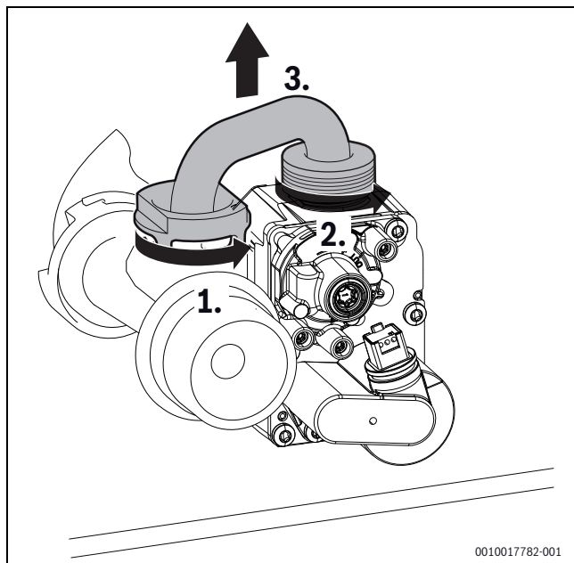
Fig. 59 Desmontar o tubo do gás
