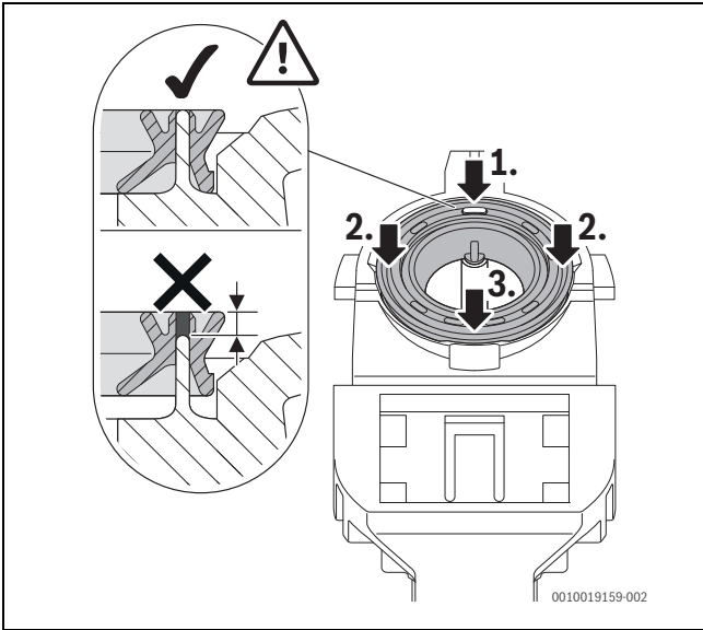
Fig. 57 Pressionar o vedante
