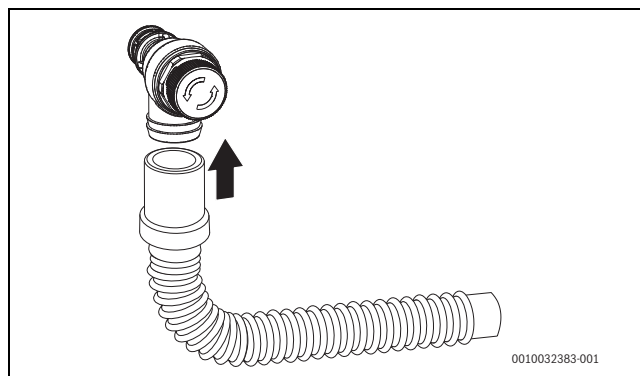
Fig. 21 Instalar a mangueira na válvula de segurança (aquecimento)
