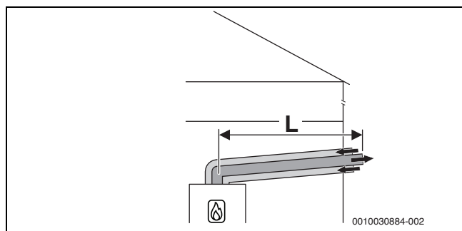
Fig. 7 Sistema de gases queimados concêntrico e horizontal de acordo com C 13x através da parede externa
