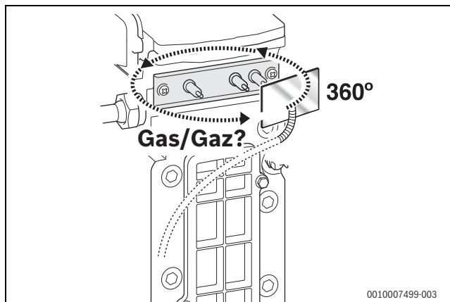
Fig. 41 Verificar a estanquidade
