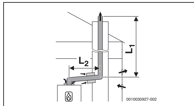
Fig. 11 Tubagem rígida de gases queimados na conduta de acordo com B_{23p}/B_{53p} com ar de admissão dependente do ar ambiente no aparelho e peça de ligação concêntrica entre o local de instalação e a conduta
