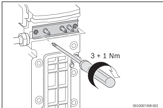
Fig. 40 Instalar o conjunto de elétrodos
