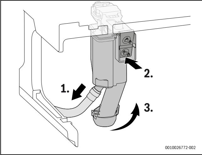
Fig. 55 Desmontar a recolha de condensados
