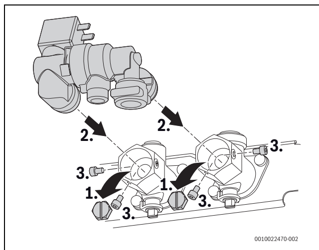
Fig. 20 Montar o dispositivo de enchimento automático
