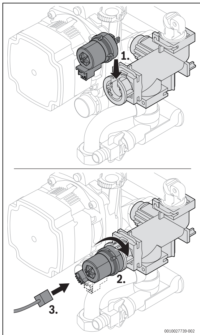
Fig. 63 Montar o motor na válvula de 3 vias (versão sem parafusos)
