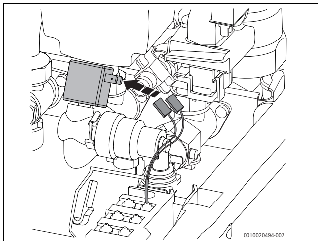
Fig. 31 Ligar o dispositivo de enchimento automático
