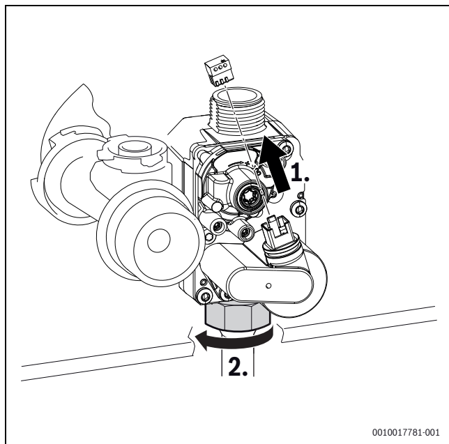
Fig. 60 Retirar a ficha e soltar a porca de aperto
