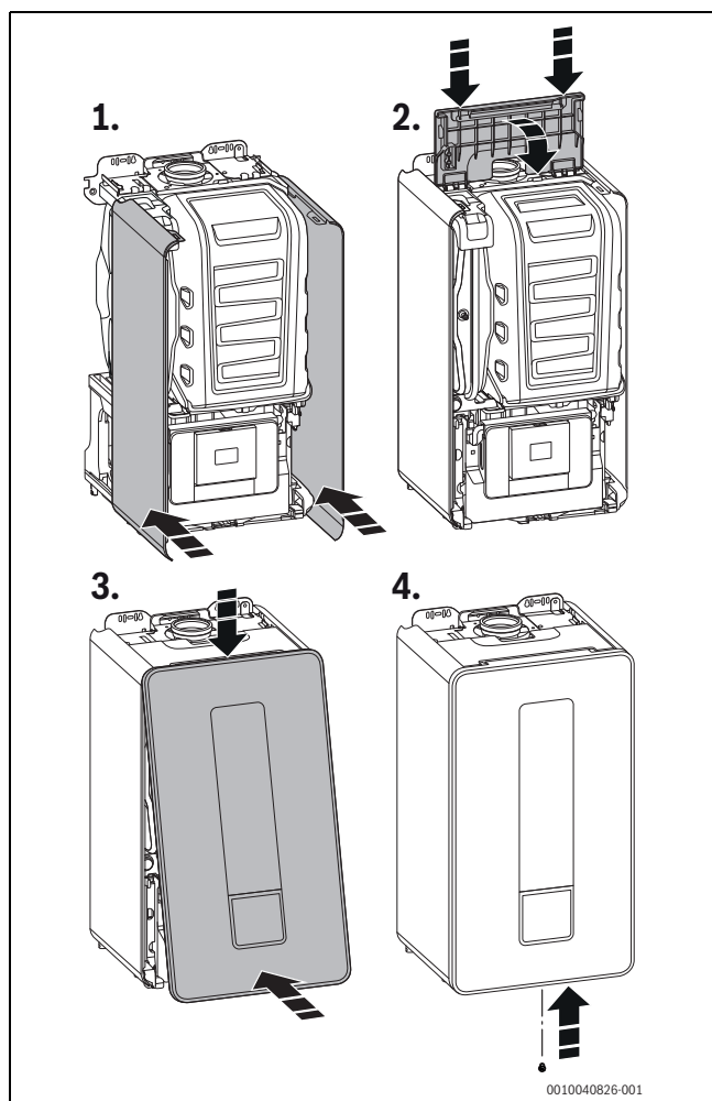
Fig. 32 Montagem do revestimento
