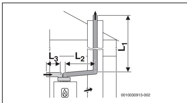
Fig. 9 Tubagem rígida de gases queimados de acordo com C_{53} na conduta e condução dos gases de escape para o exterior com tubos separados para ar de admissão e escoamento de gases queimados no local de instalação
