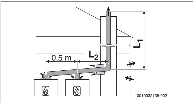
Fig. 13 Cascata com 2 aparelhos: Condução de gases queimados na conduta de acordo com B 23p /B 53p com ar de admissão dependente do ar ambiente no aparelho
