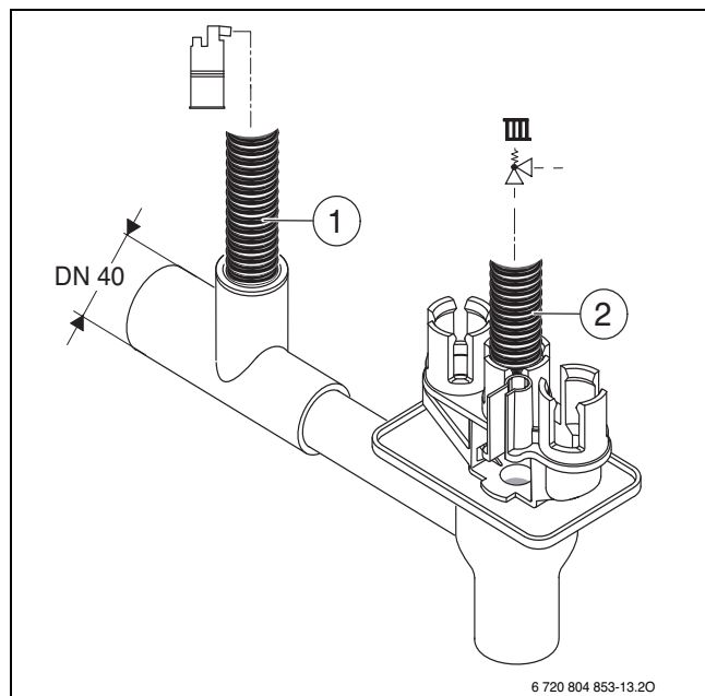
Fig. 23 Instalar a mangueira de condensados e a mangueira da válvula de segurança no sifão
