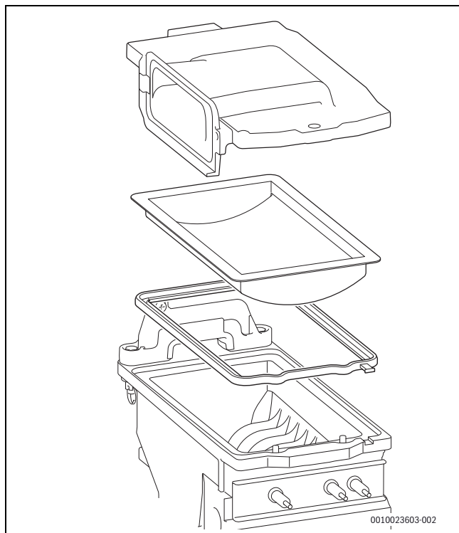
Fig. 43 Queimador
