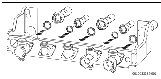
Fig. 19 Instalar os tubos com vedantes na placa de ligação para montagem
