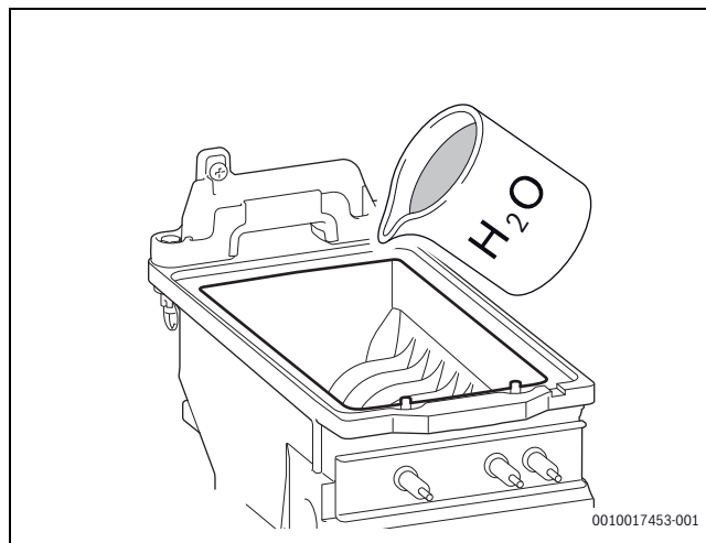
Fig. 53 Purgar o bloco térmico
