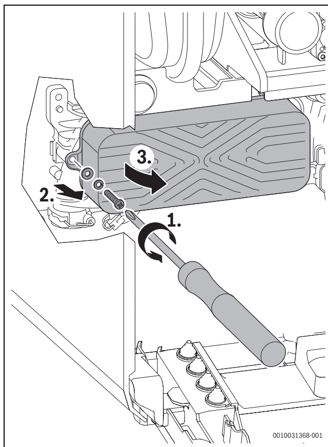
Fig. 49 Desmontar o permutador de calor de placas
