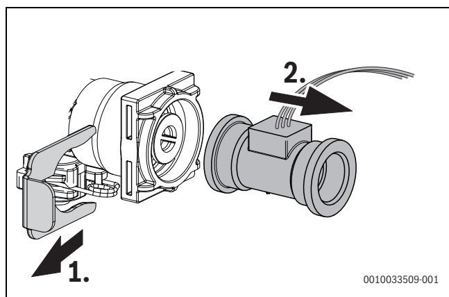
Fig. 48 Desmontar a turbina do tubo de água fria
