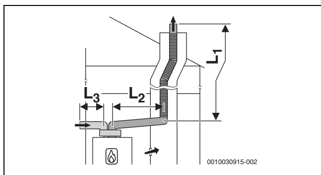
Fig. 10 Tubagem flexível de gases queimados de acordo com C_{53} na conduta e condução dos gases de escape para o exterior com tubos separados para ar de admissão e escoamento de gases queimados no local de instalação
