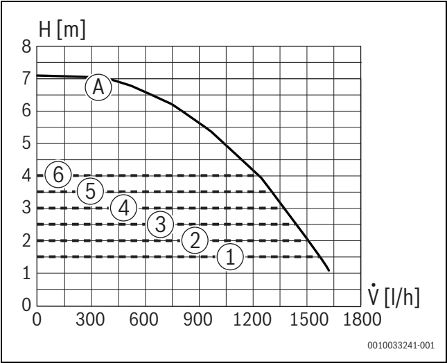
Fig. 66 Campos de funcionamento da bomba e curvas caraterísticas da bomba
