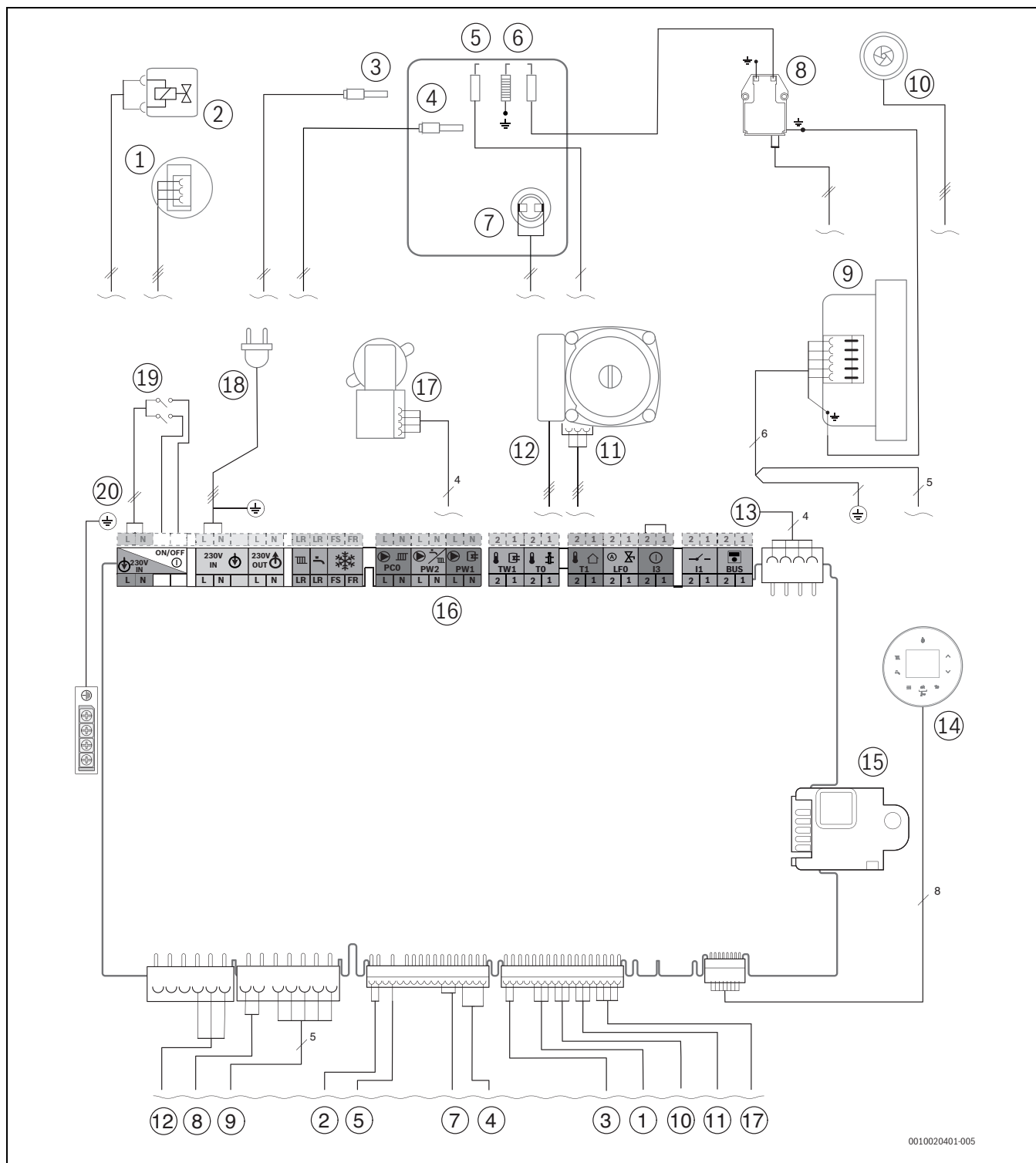
Fig. 67 Cablagem elétrica
