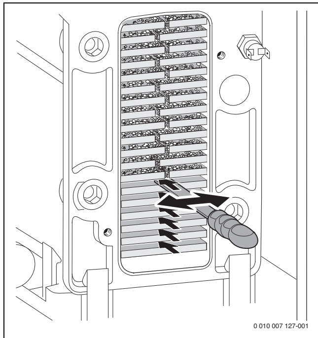
Fig. 51 Lâmina de limpeza
