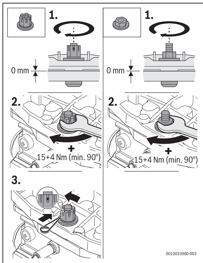
Fig. 44 Apertar a porca na tampa do queimador
