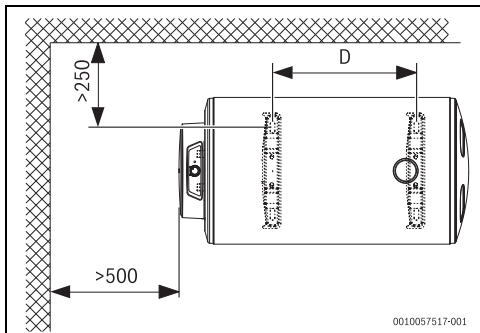
Fig. 3 Dimensões em mm (montagem mural, instalação horizontal)
