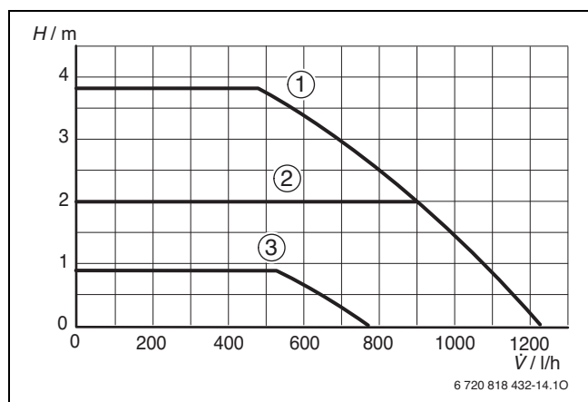
Fig. 18 Curva característica com pressão constante
