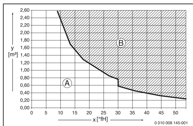
Fig. 7 Requisitos relativos à água de enchimento e à água adicional em °fH para instalações < 50 kW
