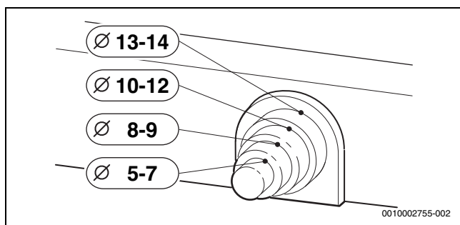
Fig. 14 Adaptar o dispositivo de redução de tração ao diâmetro do cabo
