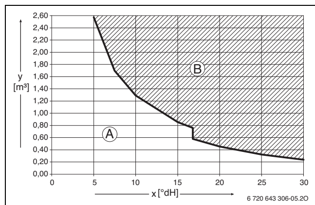
Fig. 6 Requisitos relativos à água de enchimento e à água adicional em °dH para instalações < 50 kW
