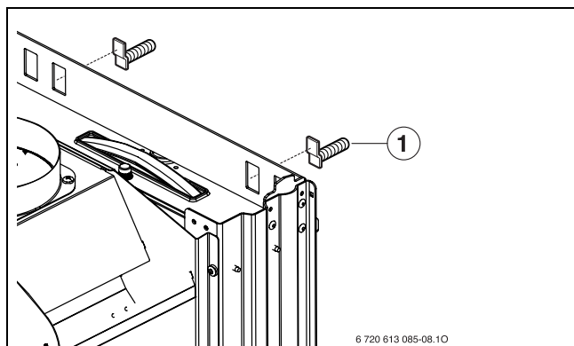
Fig. 11 Pendurar o aparelho
