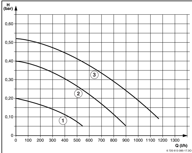
Fig. 38 Curvas características das bombas em ZWC 24/28-3, ZSC 24-3 (sem placa de ligação de montagem)
