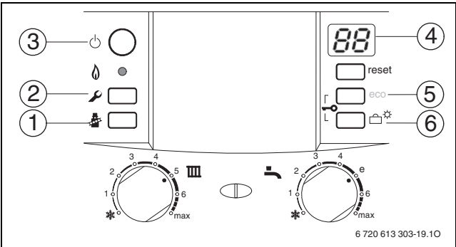
Fig. 40 Vista geral dos elementos de comando
