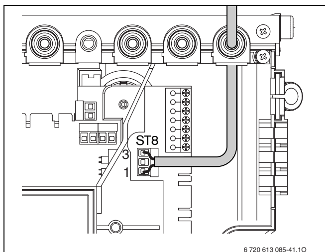
Fig. 23 Ligação do termóstato do acumulador
