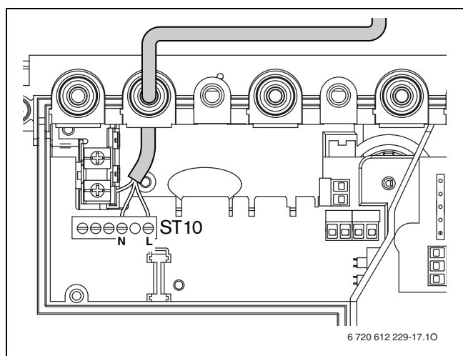
Fig. 25 Terminal de bornes, alimentação de tensão ST10
