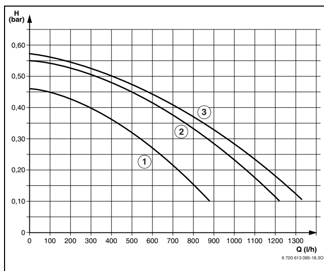
Fig. 39 Curvas características das bombas em ZWC 28/28-3, ZSC 28-3 (sem placa de ligação de montagem)
