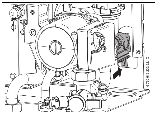
Fig. 62 Válvula de segurança (aquecimento)
