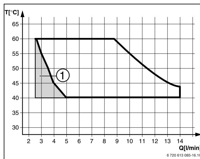
Fig. 32 Diagrama para uma temperatura de entrada da água fria de +15°C (ZWC 24/28-3..., ZWC 28/28-3...)
