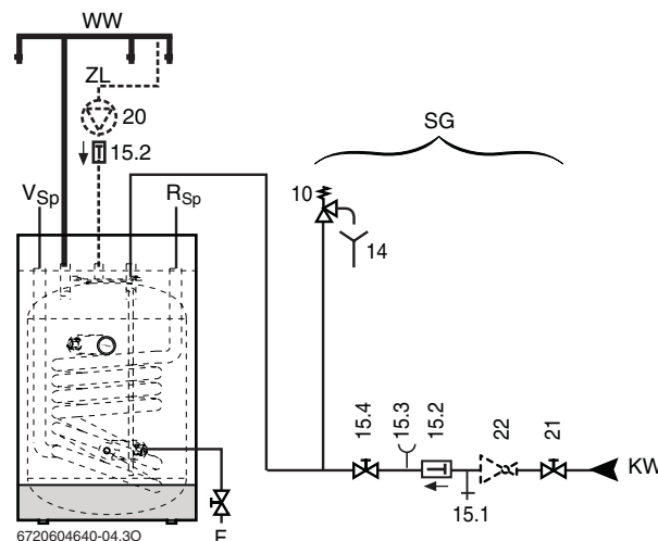
Fig. 4 Esquema de conexões pelo lado da água sanitária
