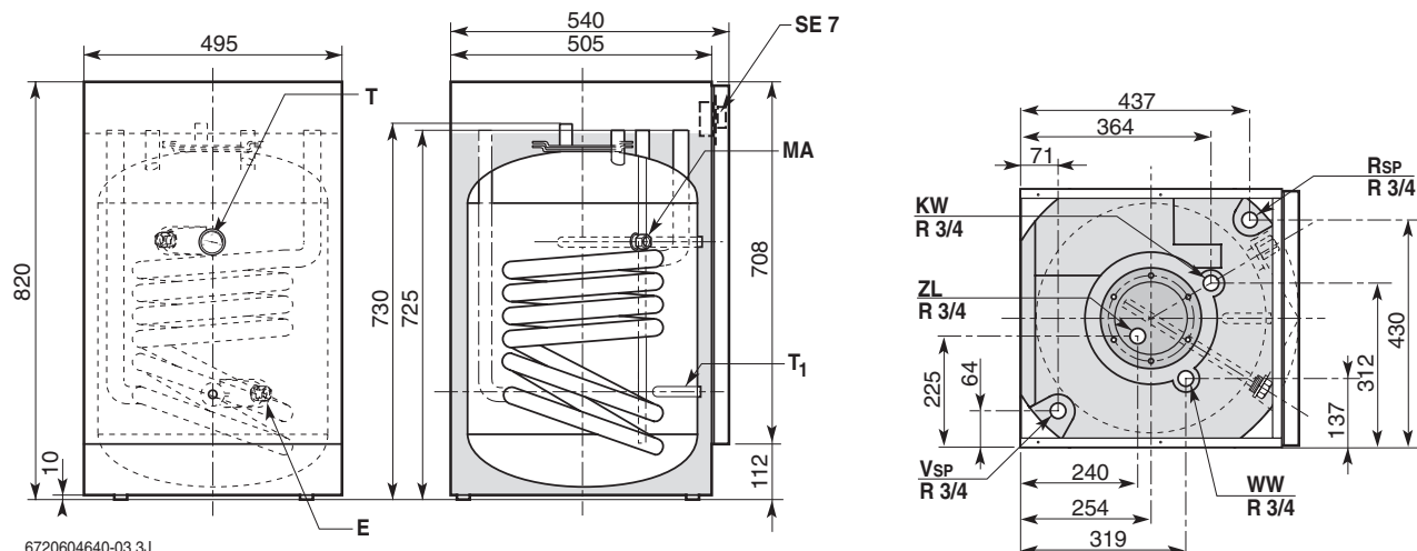
Fig. 1 Visto por cima, sem tampa
