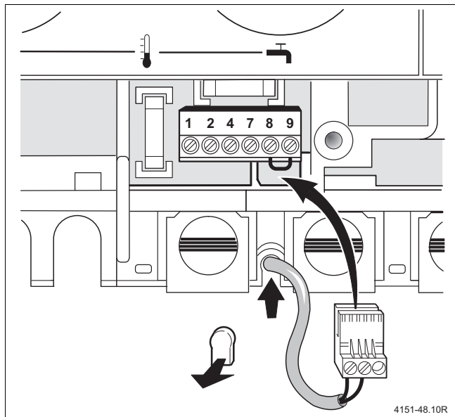
Fig. 5 Introduzir a ficha
