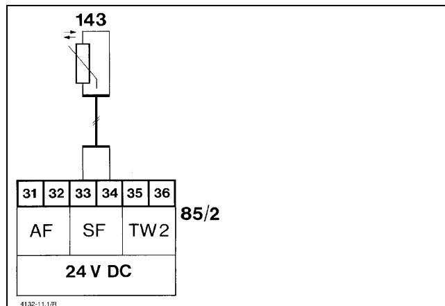
Fig. 7 Ligação do sensor de temperatura do acumulador
