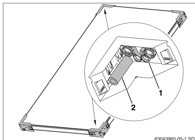
Fig. 4 Dois cantos de transporte com um conjunto de união
