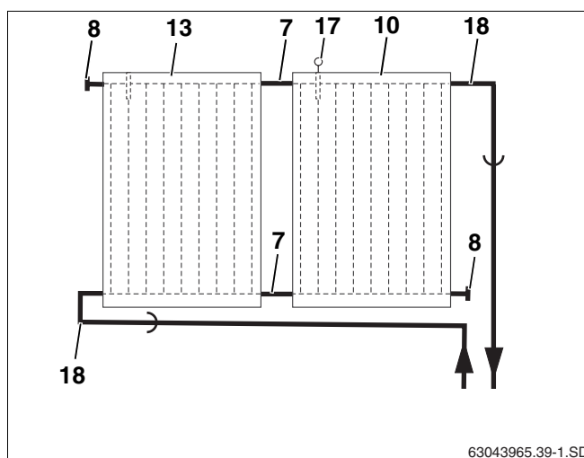
Fig. 62 Ligação hidráulica
