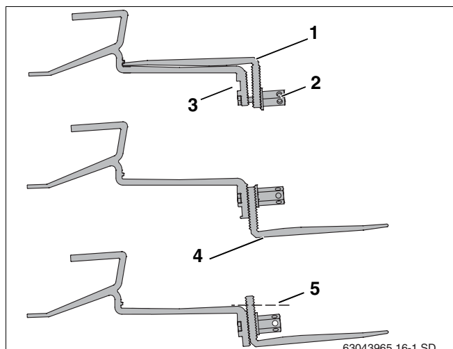
Fig. 14 Fixar o gancho para telhados ao caibro
